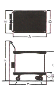
■寸法図(ASP-300-T2)
